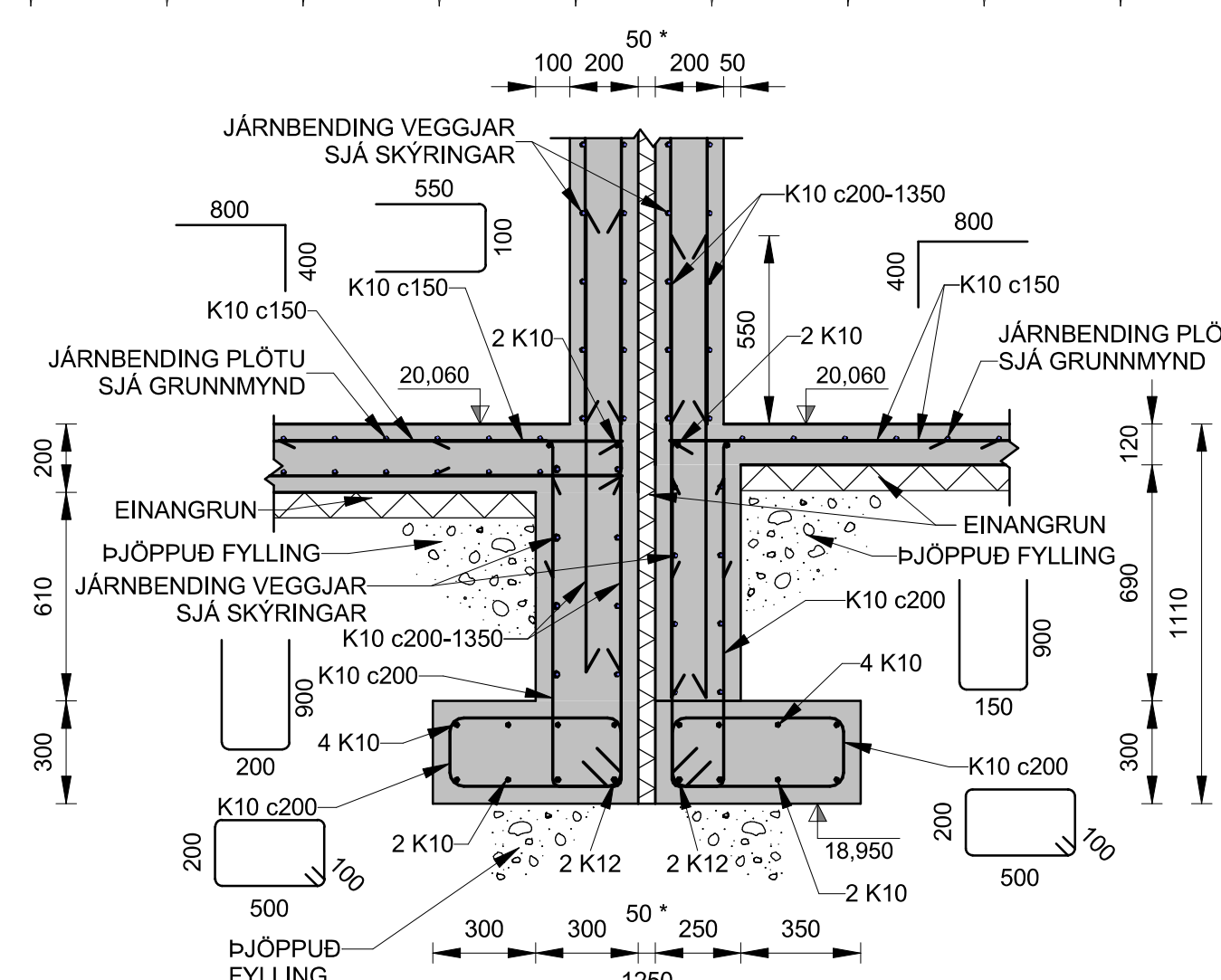
U017 SNIE G003 1 : 20 G004 G103 G104
