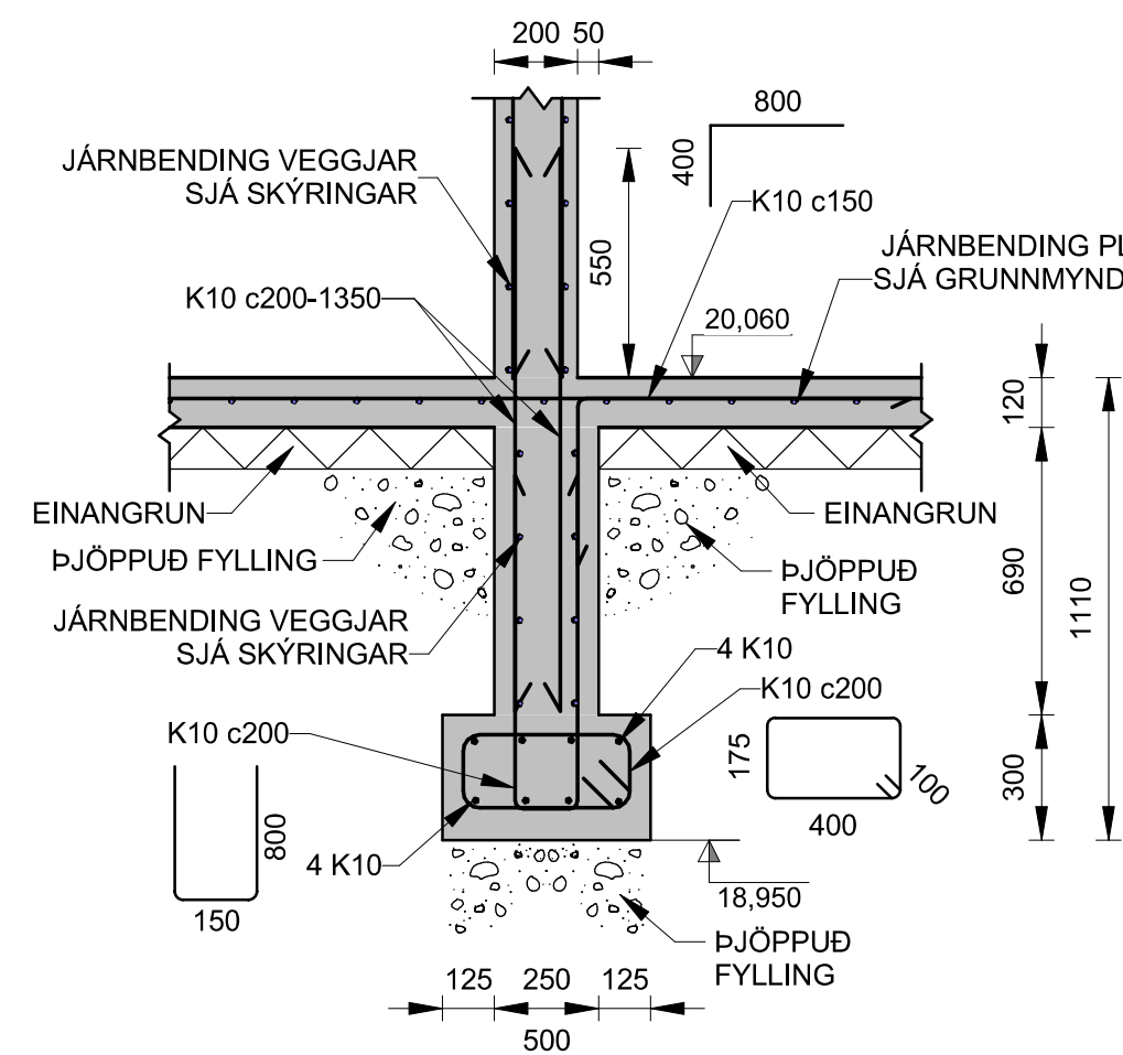
U014 SNID G002 1 : 20 G102
