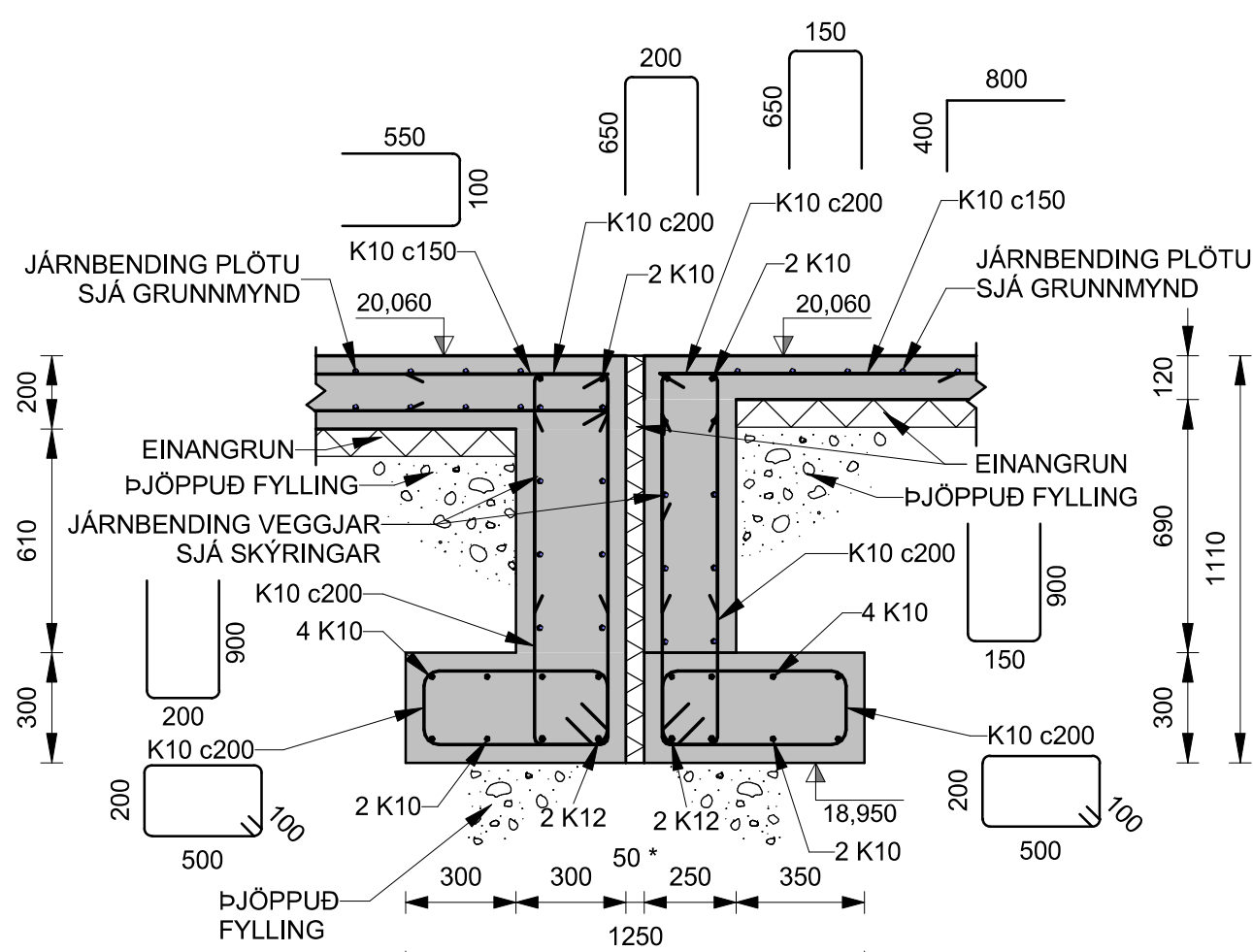
U016 SNID G003 1 : 20 G004 G103 G104
