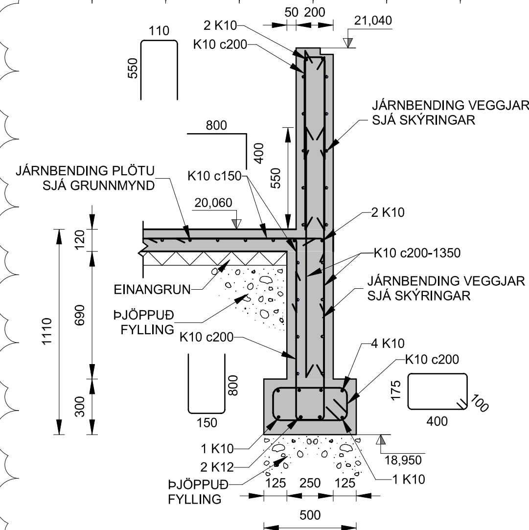
U015 SNID G001 1 : 20 G101
