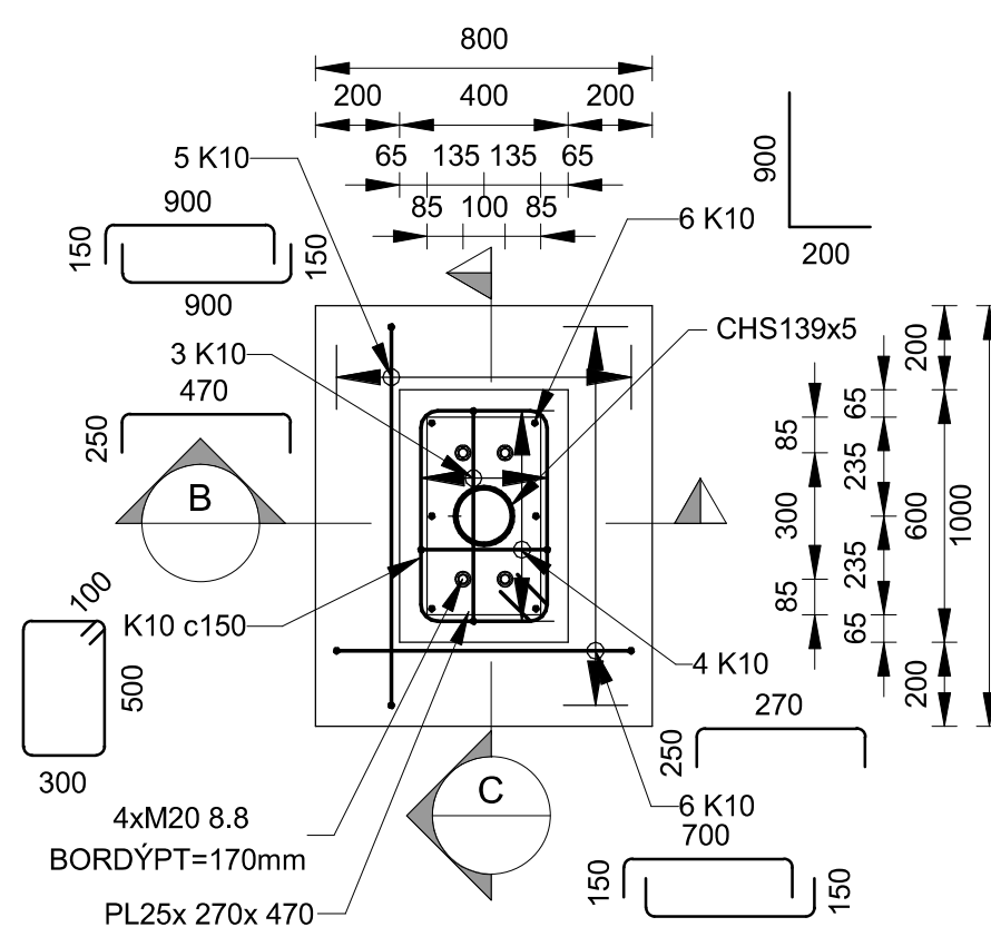
U019 DEIL G001 1 : 20 G004
