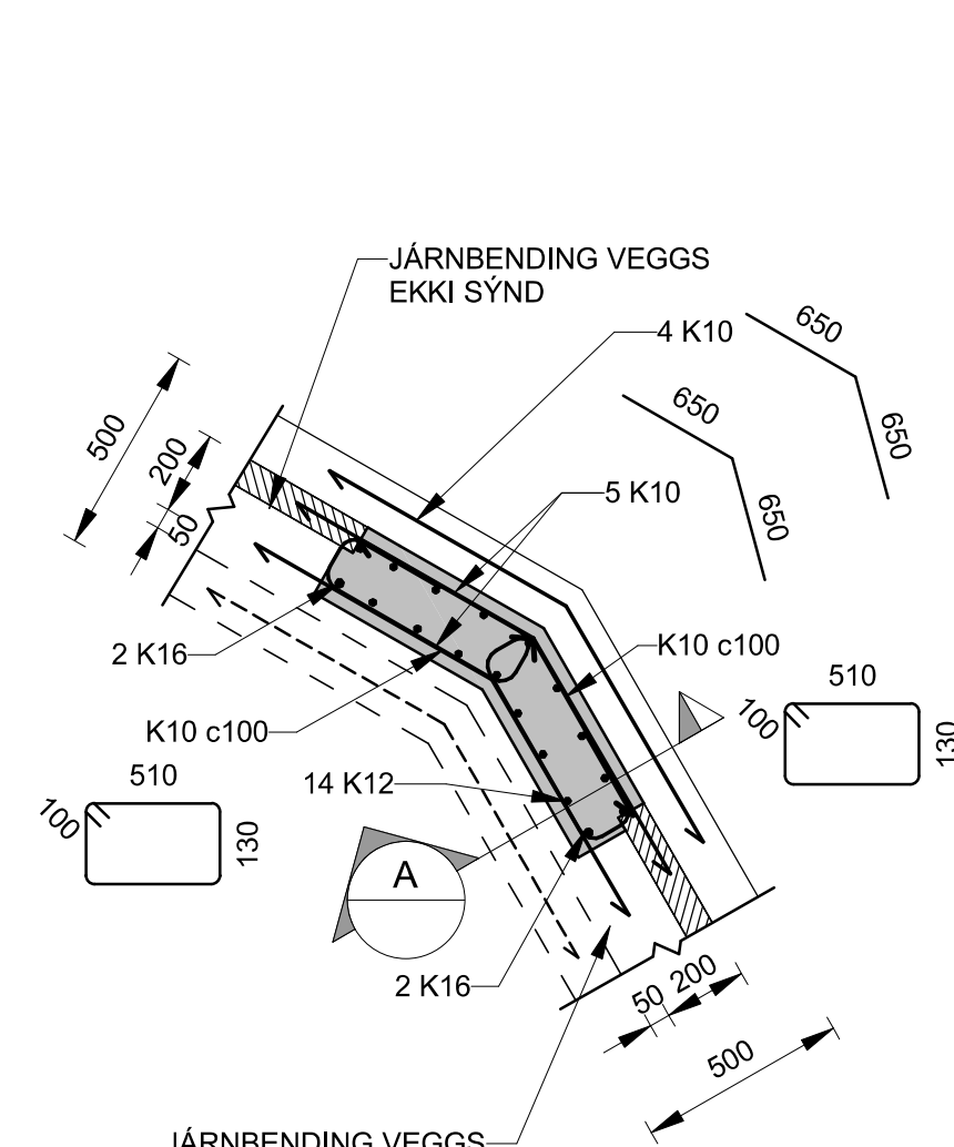
U018 DEIL G103 1 : 20
